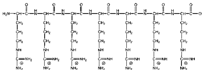
Arg7
