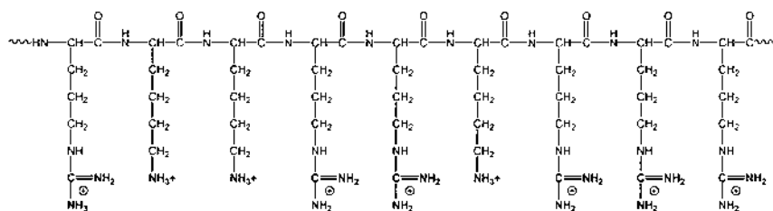
Tat 49-57
